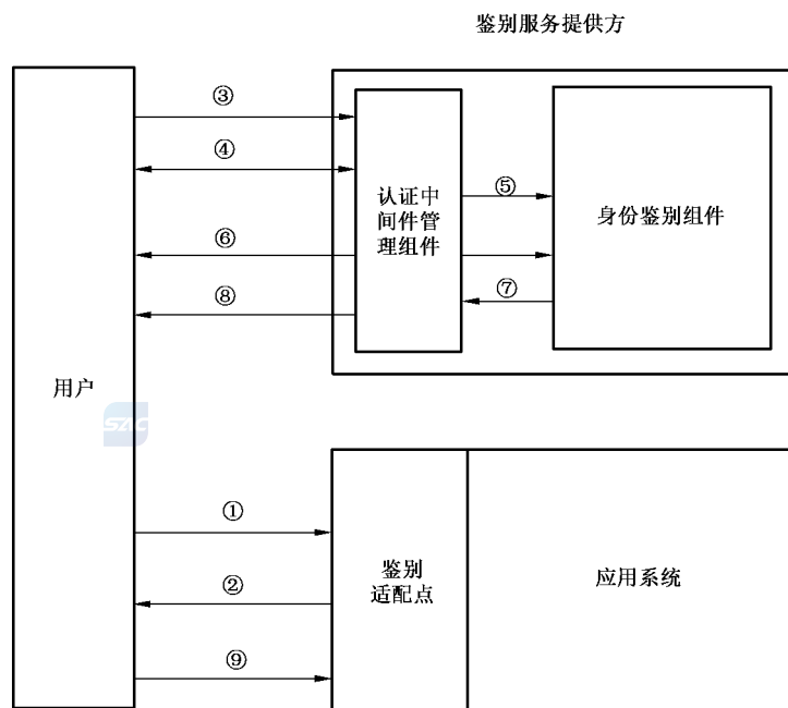
图 A.1 直接鉴别模式下的身份鉴别流程
