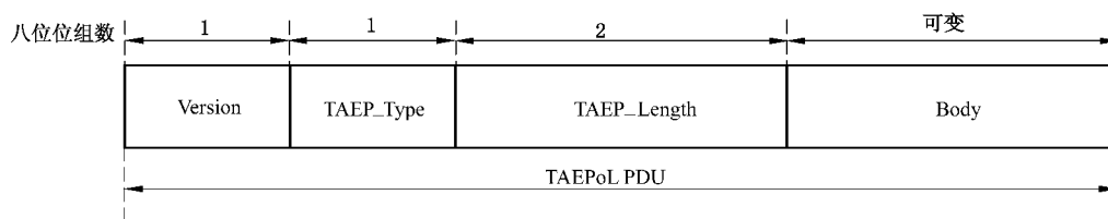
图 D. 39 TAEPoL PDU 的格式
