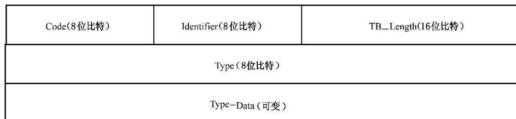
图 D.41 Request 和 Response 类型的 TAEP 分组格式示意图
