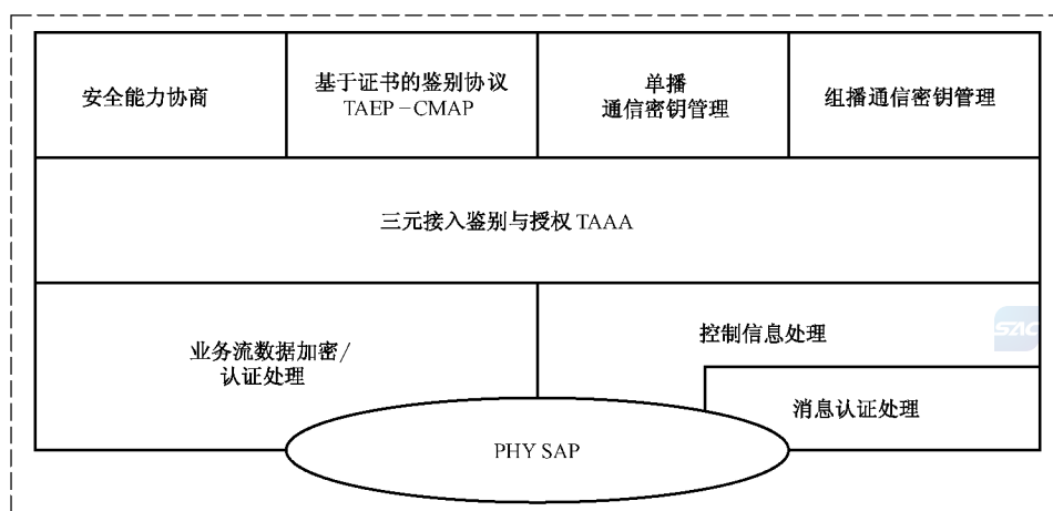
图 C.1 安全子层
