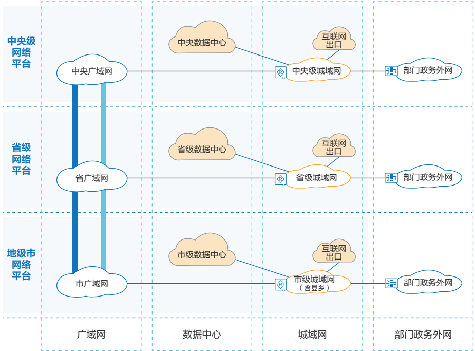
图3-1 电子政务外网架构
